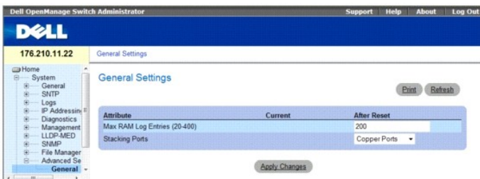
Рис. 6-111. Страница General Settings (Общие параметры)
