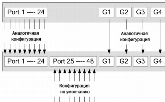
Рис. 1-5. Замещение порта коммутатора PowerConect 3548/P портом коммутатора PowerConnect 3524/P
