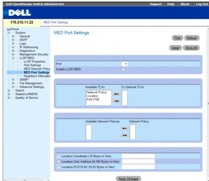
Рис. 6-82. MED Port Settings (Параметры MED для порта)
