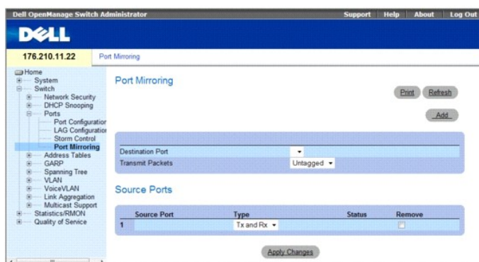
Рис. 7-27. Страница Port Mirroring (Зеркалирование портов)
